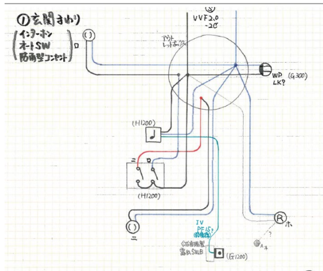
図4 複線図(一部抜粋)
